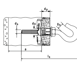
Fissaggio basculante in nylon fischer DUOTEC 12 H con gancio M6
